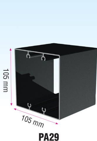
Encombrement version façade
